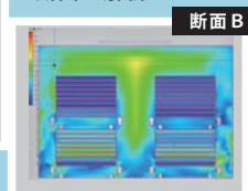
断面 B
